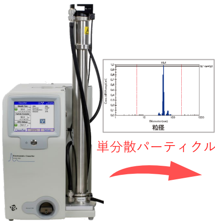
静電分級器 (DMA) Model : 3082
